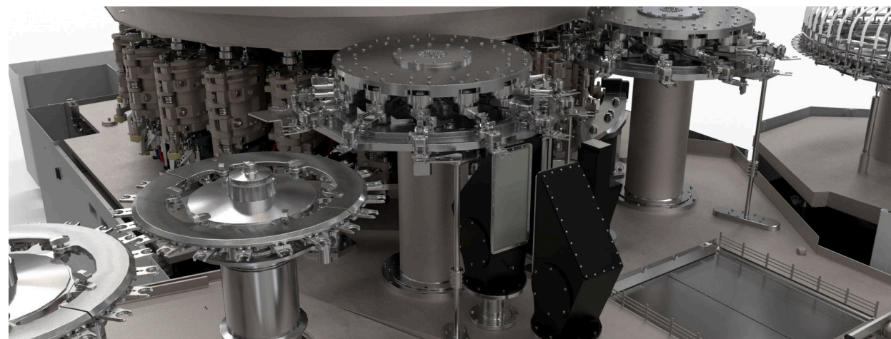
Contipure AseptBloc 内的轮廓和侧壁检测
